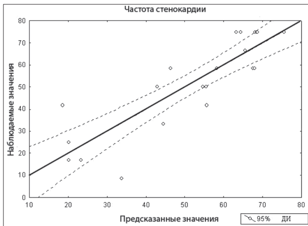
Рис. 1. Частота стенокардии. Линейная регрессия — предсказанные значения против наблюдаемых.
